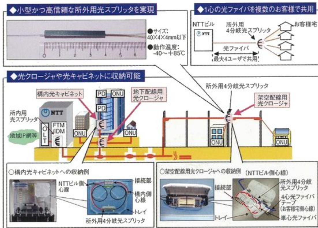
図 所外用光スプリッタとその収納技術
