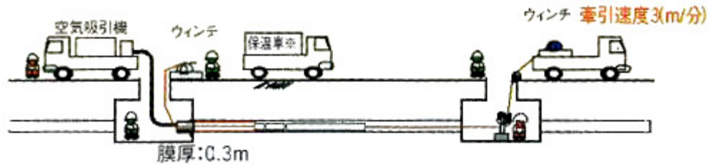
図 負圧式ライニング技術
