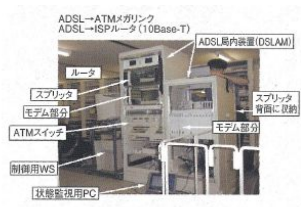
図 ADSL フィールド実験
